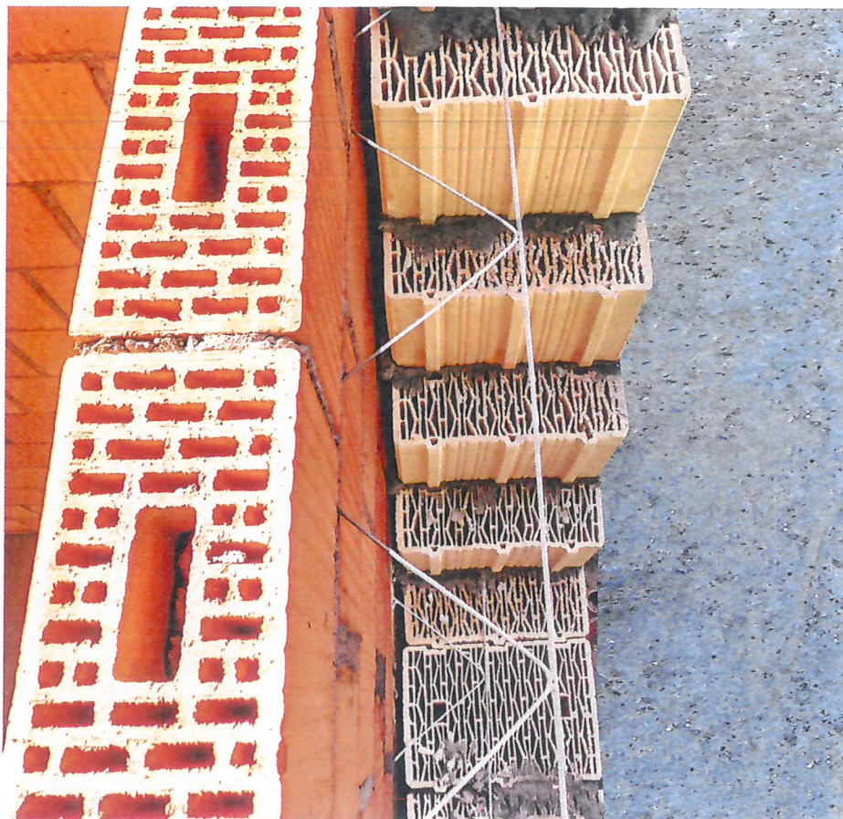
Das ökologische Backsteinsystem verbindet Dämm- und Tragfunktion.
